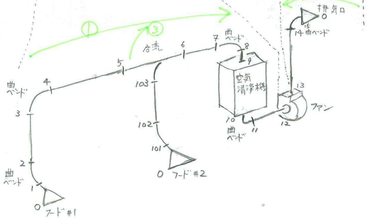
系統線図
