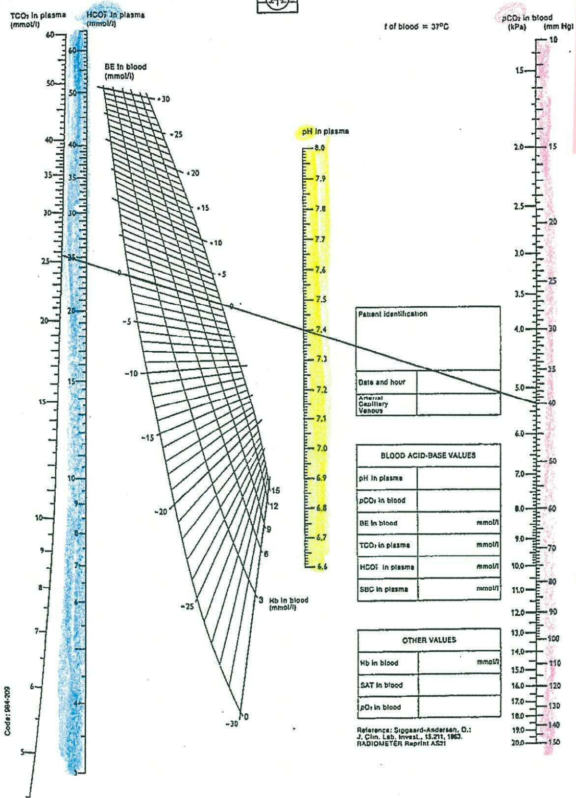
図3 Siggaard-Andersen Alignment Nomogram 図中に正常値の位置を示してある。
