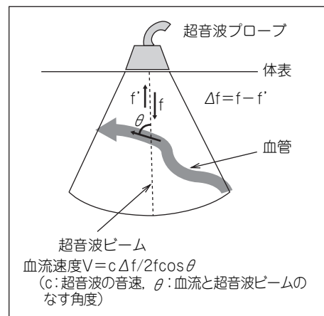
(図 C-15-1) パルスドップラー法の原理
