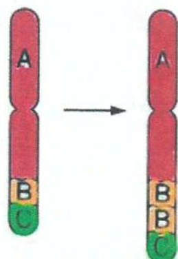
8. 重複
