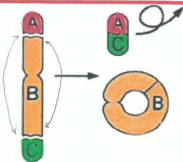
6. 環状染色体
