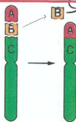
5. 欠失
