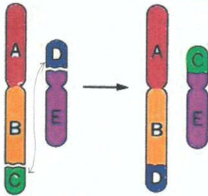
1. 転座
