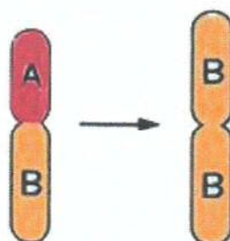
7. 同腕染色体
