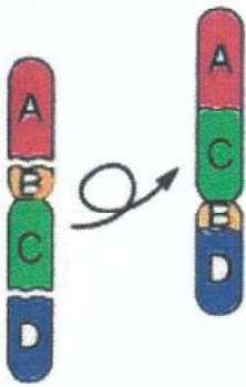
3. 逆位
