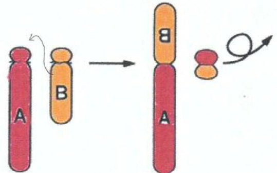
2. Robertson型転座
