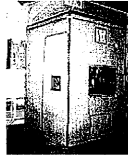
自動打ち抜きプレス FC#7000 減音量 15dB(A)
