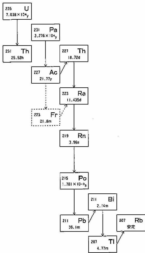
アクチニウム系列 (4n+3) 系列
