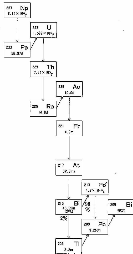
ネプツニウム系列 (4n+1) 系列
