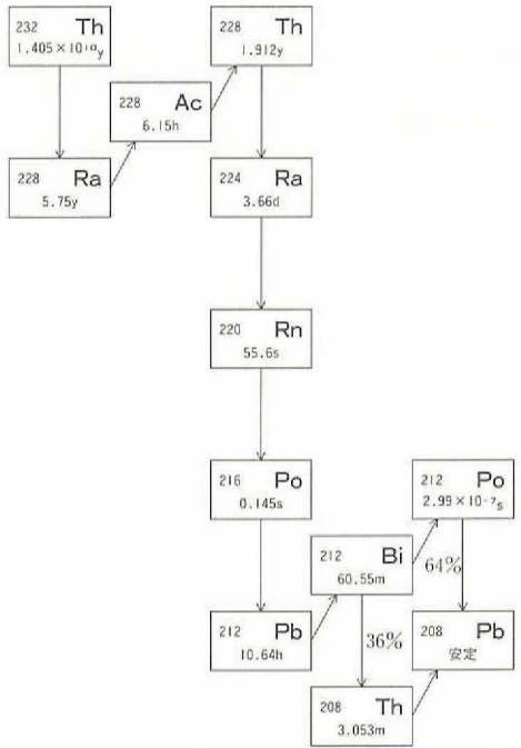
トリウム系列 4n 系列
